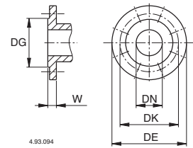
Flanges PN 10, EN 1092-2
