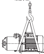
Fig. 7 Sollevamento pompa Raising the pump Anhebung Pumpe Suolèvement de la pompe Elevación de la bomba 吊起水泵
