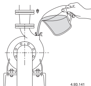
Abb. 3 Auffüllung.
