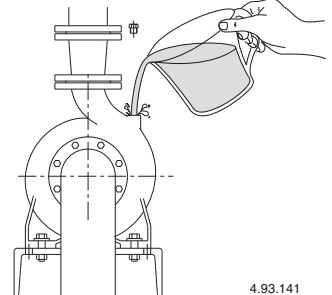
Fig. 3 Cebado.
