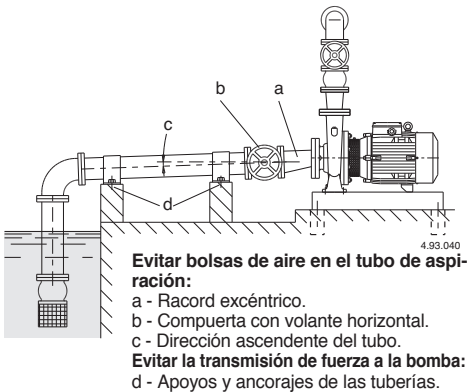
Fig. 2 Montaje y unión de la instalación de los tubos.
