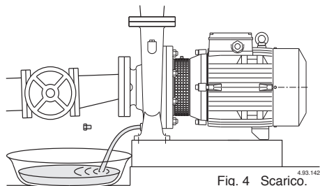
Fig. 4 Scarico.
