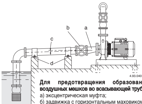
Рис. 2 Подсоединение труб
