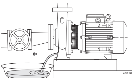
Рис. 4 Слив воды
