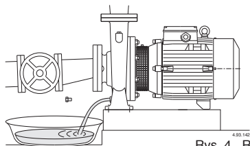
Rys. 4 Rozładunek.
