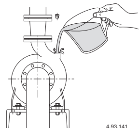
Σχ. 3 Πλήρωση
