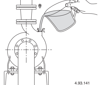
Рис. 3 Заполнение жидкостью
