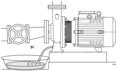
Fig. 4 Vidange.
