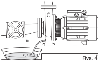
Rys. 4 Rozładunek.
