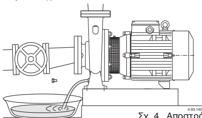
Σχ. 4 Αποστράγγιση
