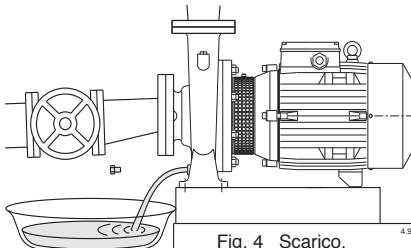
Fig. 4 Scarico.
