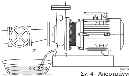
Σχ. 4 Αποστράγγιση
