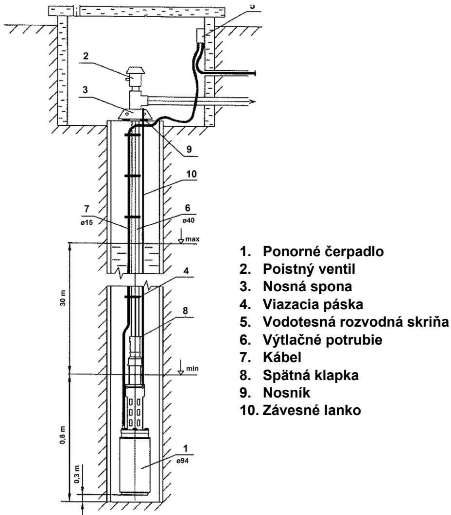
Hlavná časť čerpaceho zariadenia a montáž čerpadla do vrtu
