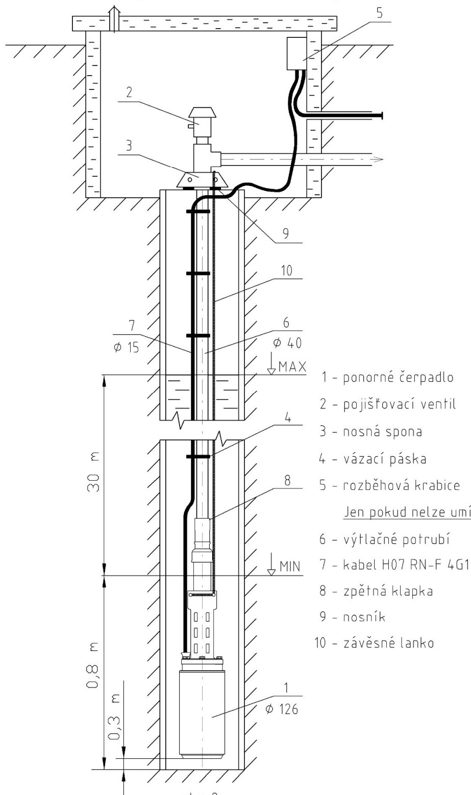
Hlavní části čerpacího zařízení a montáž čerpadla do vrtu
