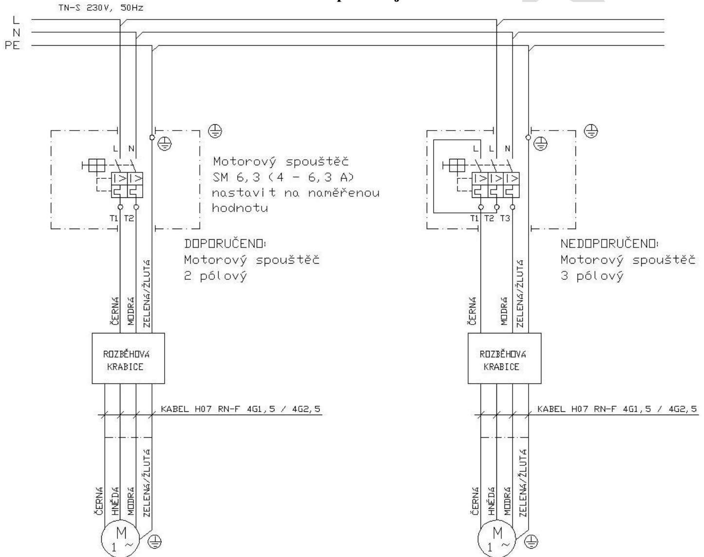
Schéma zapojení motorového spouštěče s čerpacím agregátem obr. 8
