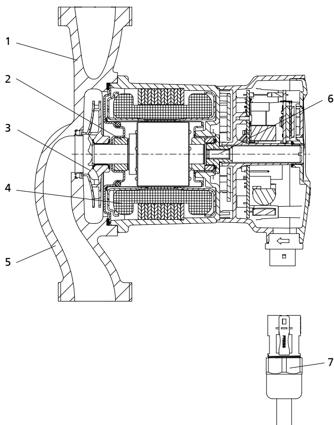
Obr. 3: Řez čerpadlem
