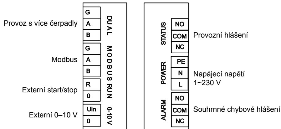
Obr. 10: Schéma zapojení typů Calio 40-120/-180, 50-100/-120/-150/-180
