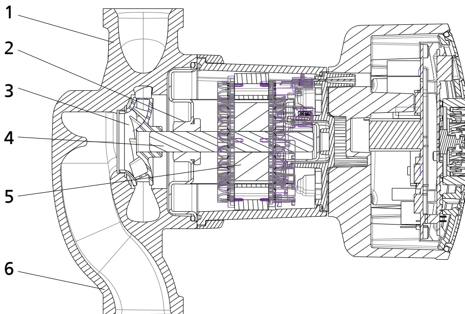
Obr. 5: Řez čerpadlem
