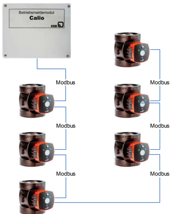
Obr. 11: Správně: položení sběrníkových kabelů v přímce
