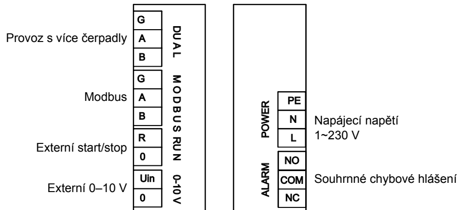
Obr. 9: Schéma zapojení typů Calio 25, 30, 32, 40-60/-70/-80/-90, 50-40/-60/-80/-90
