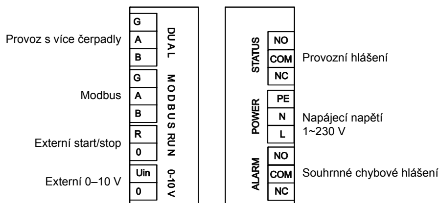
Obr. 34: Schéma elektrického zapojení typů Calio 40-120/180, 50-100/-120/-150/-180
