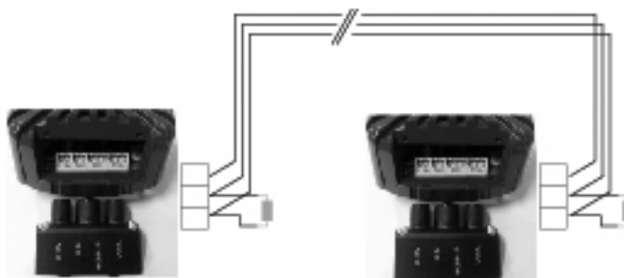
Obr. 12: Zakončovací odpory
