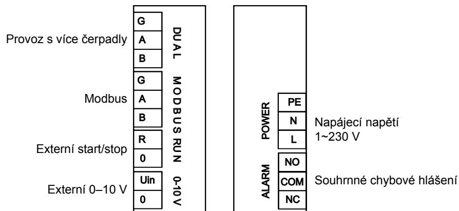
Obr. 33: Schéma elektrického zapojení typů Calio 25, 30, 32, 40-60/70/80/90, 50-40/-60/-80/-90
