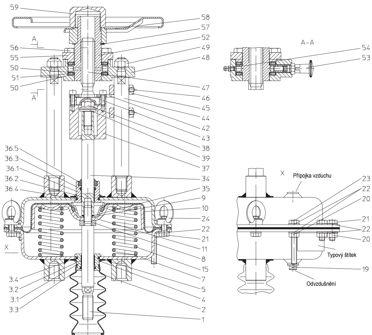
Obrázek 4: DP32 s ručním nouzovým posuvem „Hnací vřeteno zasouvané působením pružin“
