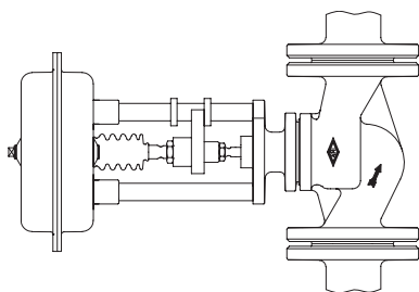
Obr. 14: Potrubí svislé
