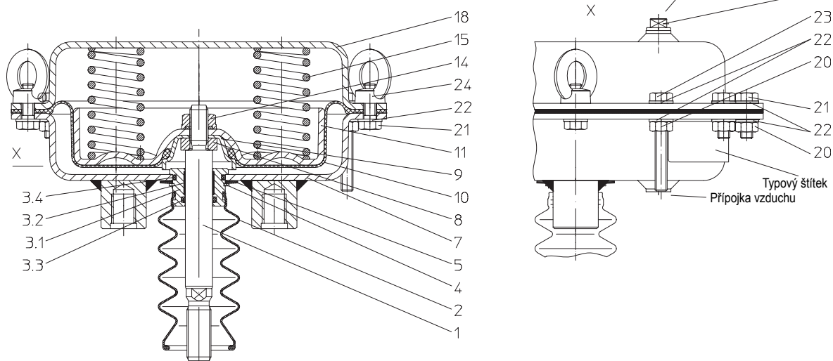
Obrázek 1: DP32 „Hnací vřeteno vysouvané působením pružin“
