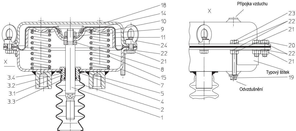
Obrázek 3: DP32 „Hnací vřeteno zasouvané působením pružin“
