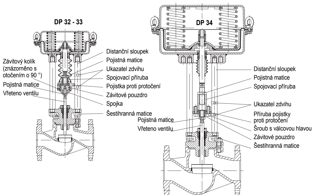
Obrázek 16: Pneumatický ovládací ventil – průchozí
