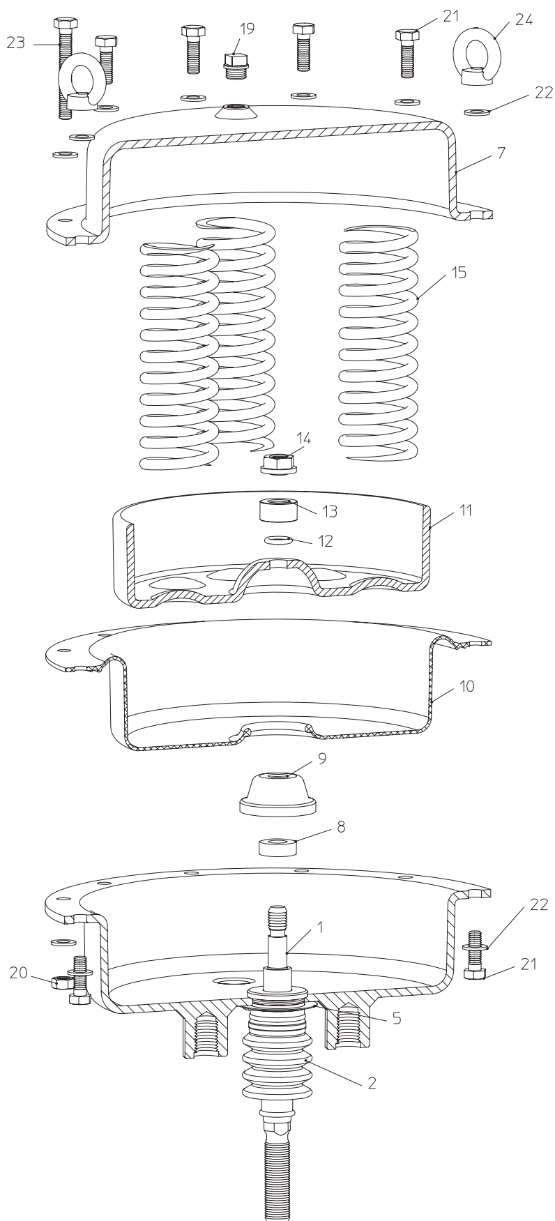
Obrázek 27: DP 33 „Hnací vřeteno vysouvané působením pružin“
