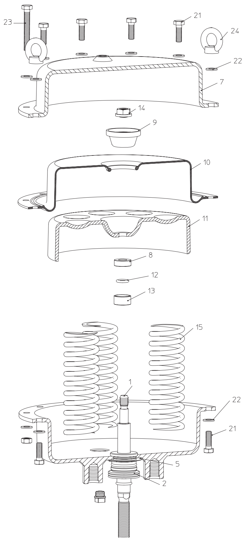
Obrázek 28: DP 33 „Hnací vřeteno zasouvané působením pružin“
