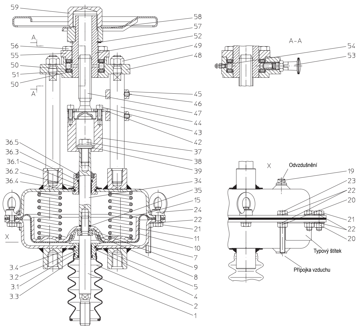
Obrázek 2: DP32 s ručním nouzovým posuvem „Hnací vřeteno vysouvané působením pružin“
