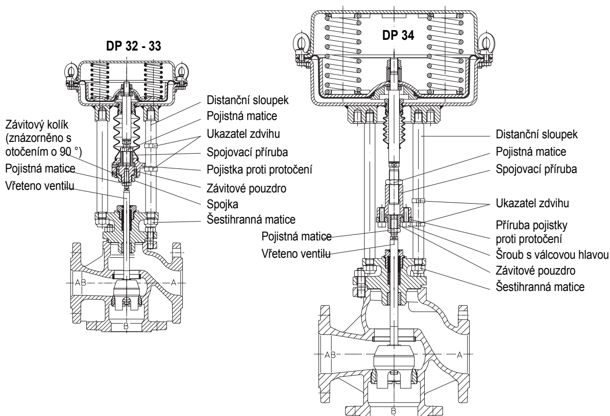
Obrázek 17: Pneumatický ovládací ventil - trojcestný směšovací ventil (průtok AB-B)
