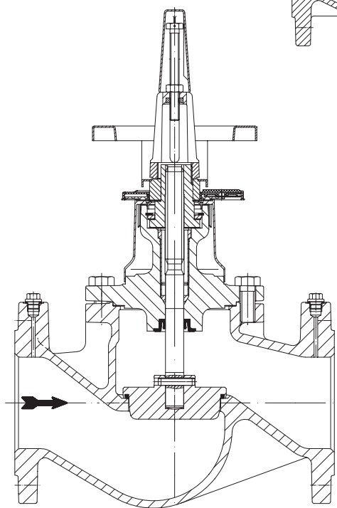
DN 100 - 200
