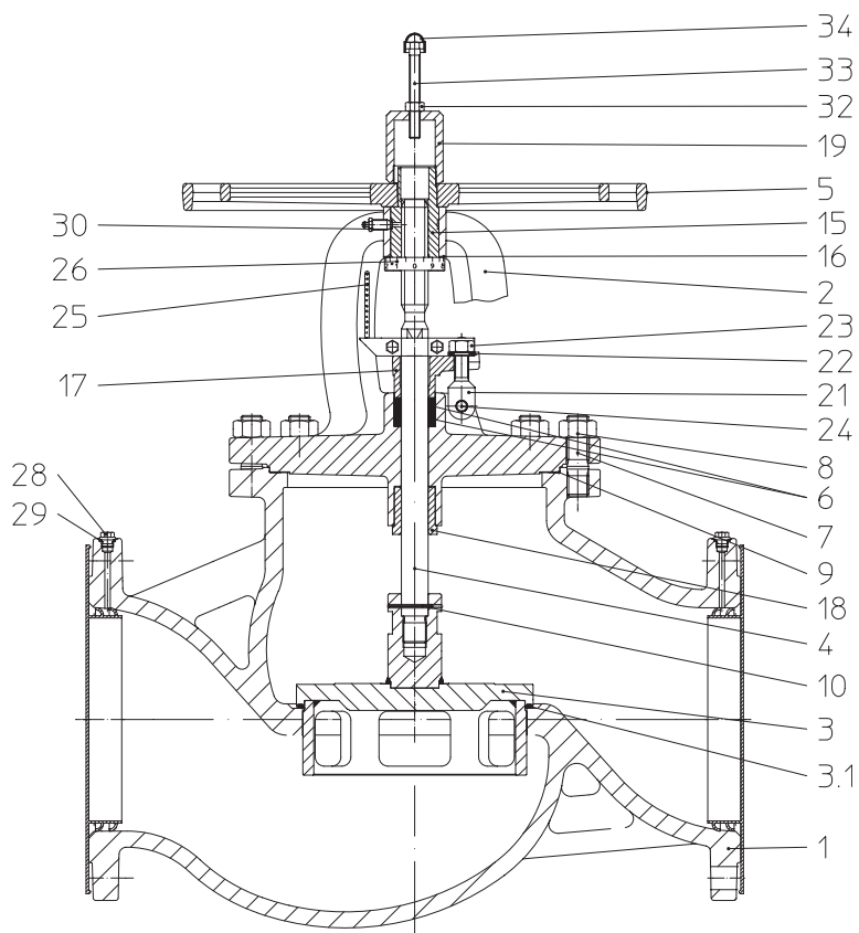
Obr. 4: DN 250-400 s horním dílem ucpávky a stupnicí zdvihu
