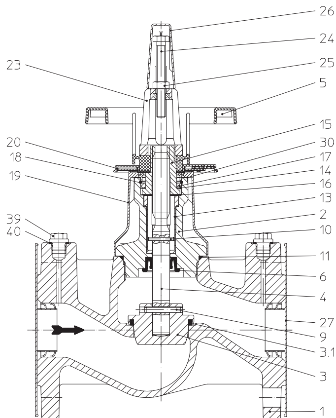
Obr. 3: DN 15 - 200 s číslicovým ukazatelem
