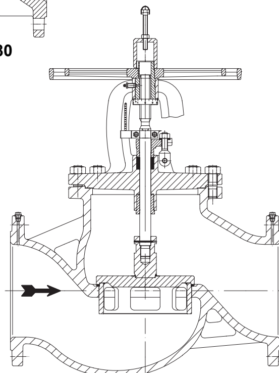
DN 250 - 400
